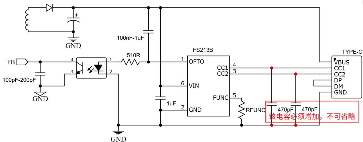
图2. FS213B应用图
