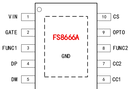
图 1. 引脚定义
