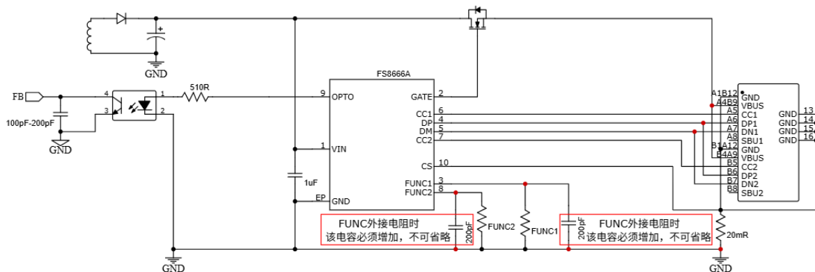
图2. FS8666A直驱光耦应用图
