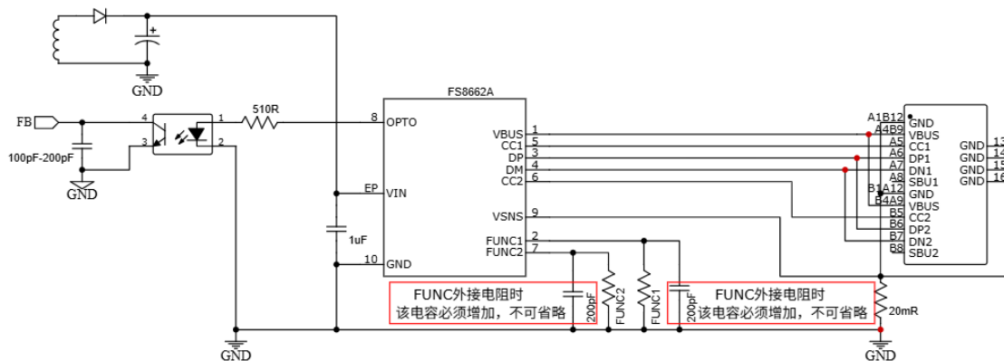
图2. FS8662A直驱光耦应用图
