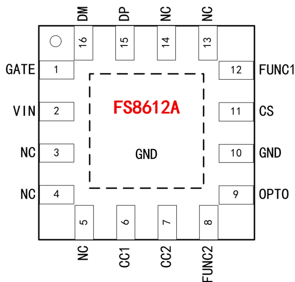
图 1. 引脚定义
