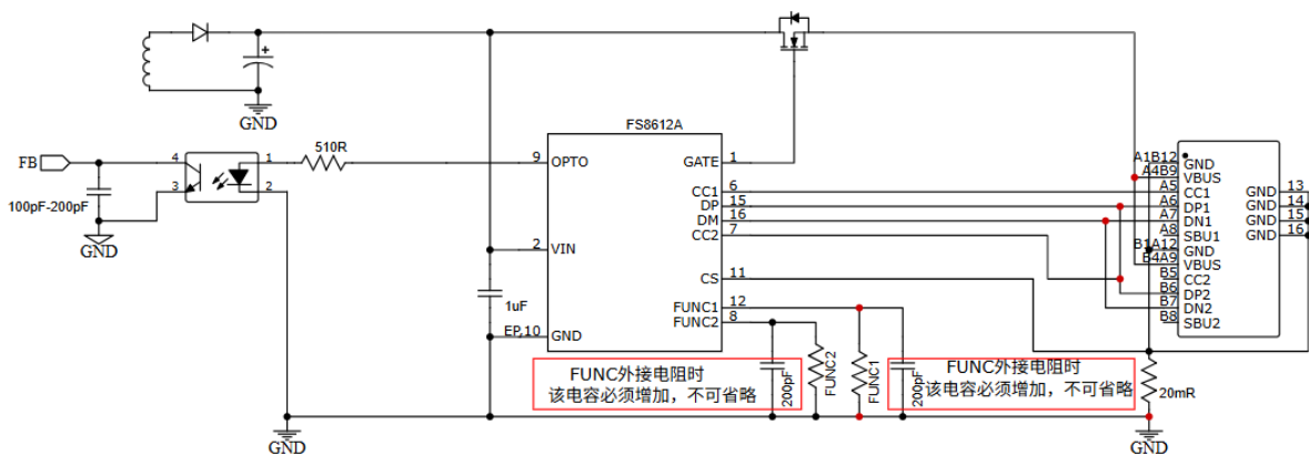
图2. FS8612A直驱光耦应用图
