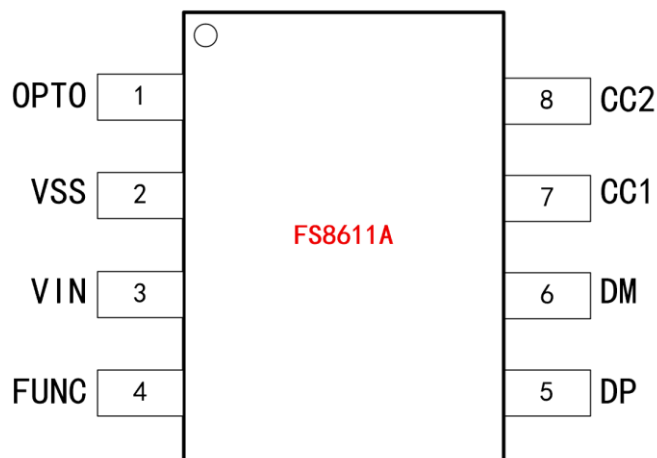
图 1. 引脚定义
