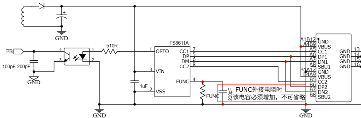
图2. FS8611A直驱光耦应用图
