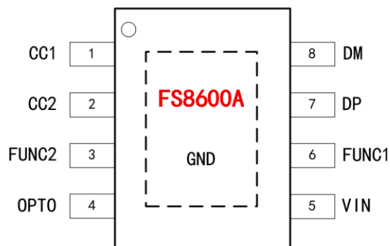
图 1. 引脚定义
