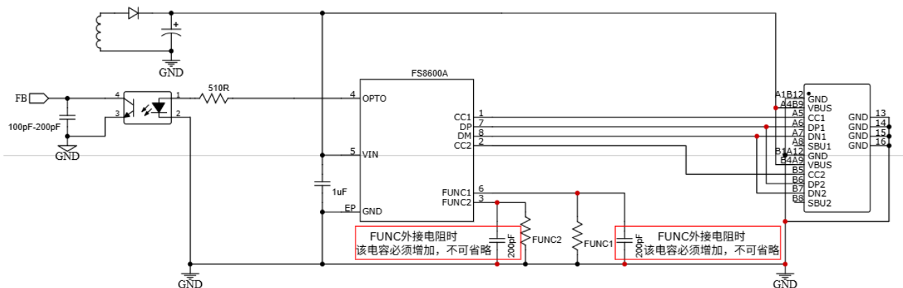
图2. FS8600Ax直驱光耦应用图
