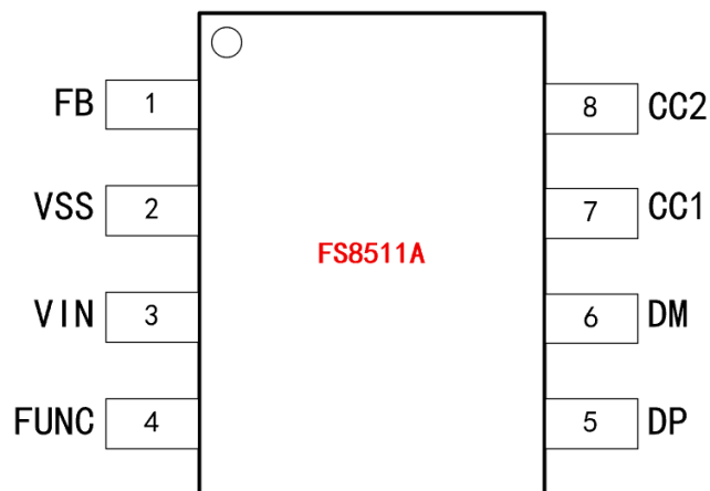
图 1. 引脚定义
