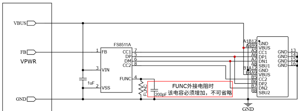
图2. FS8511A直驱光耦应用图
