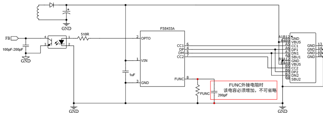
图2. FS8433A直驱光耦应用图
