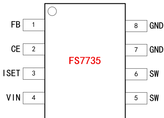
图 2. 引脚定义
