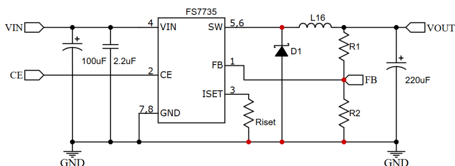
图1. 应用图
