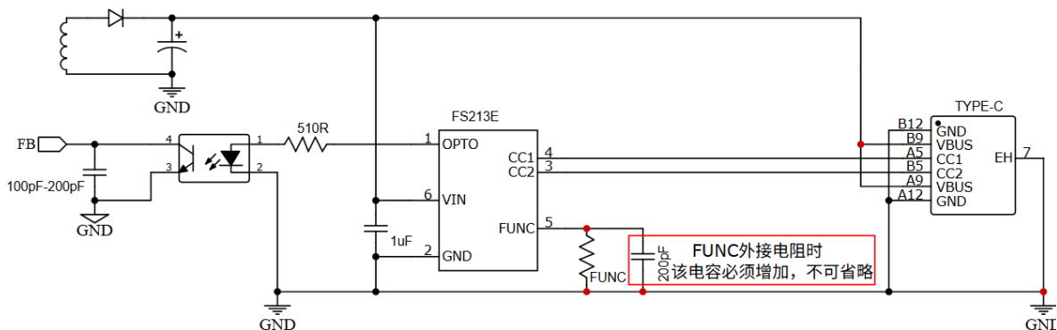
图2. FS213E直驱光耦应用图
