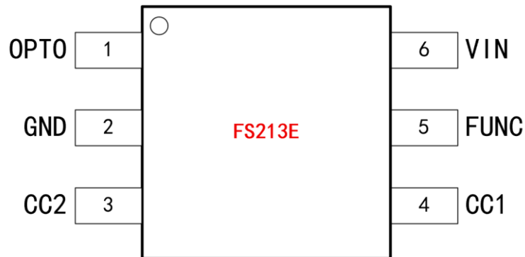
图 1. 引脚定义
