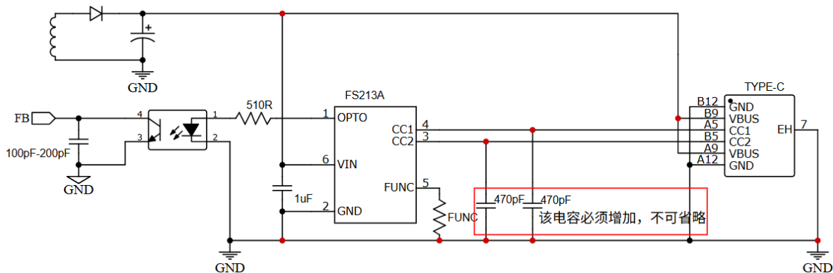
图2. FS213A直驱光耦应用图
