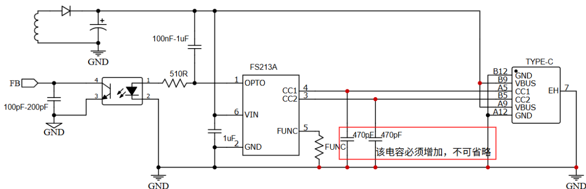
图3. FS213A模拟MOS应用图
