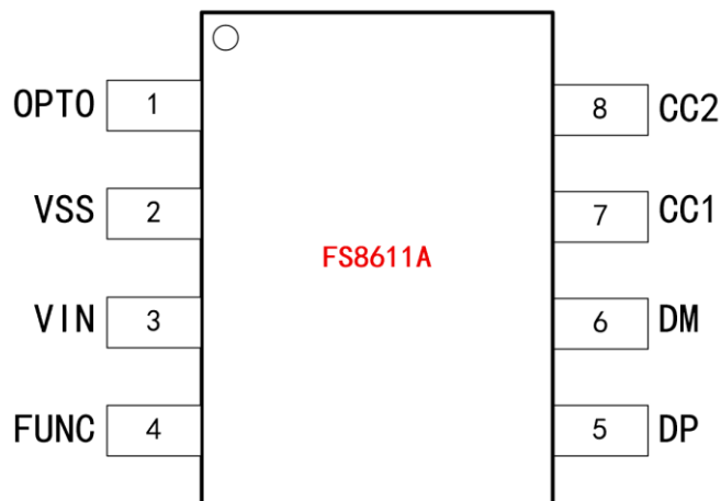
图 1. 引脚定义
