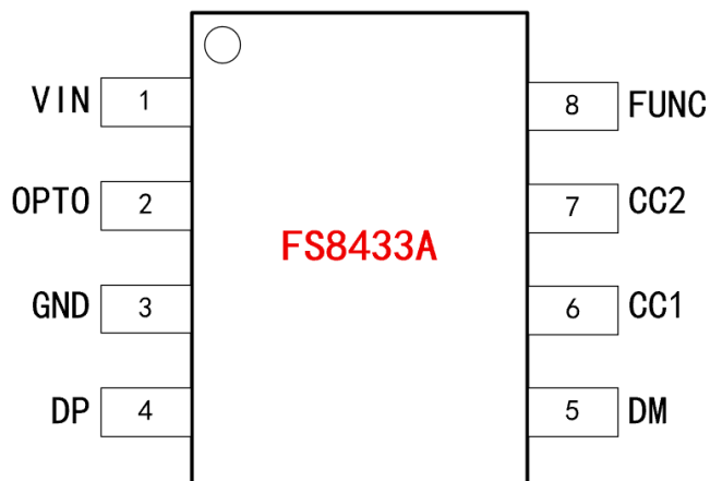
图 1. 引脚定义
