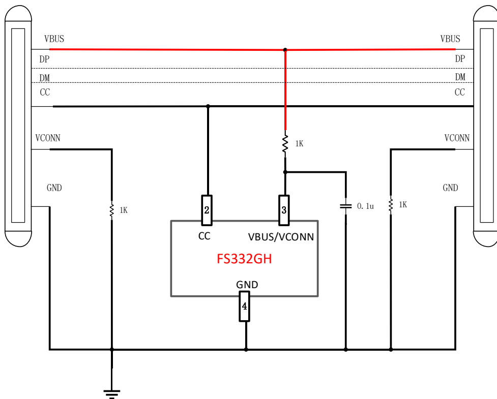
FS332GH 5芯线单芯片应用图
