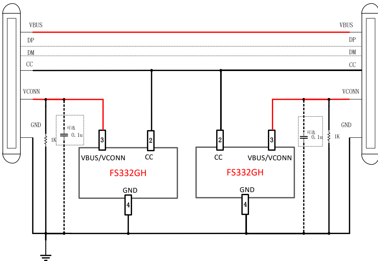
FS332GH 5 芯线双芯片应用图
