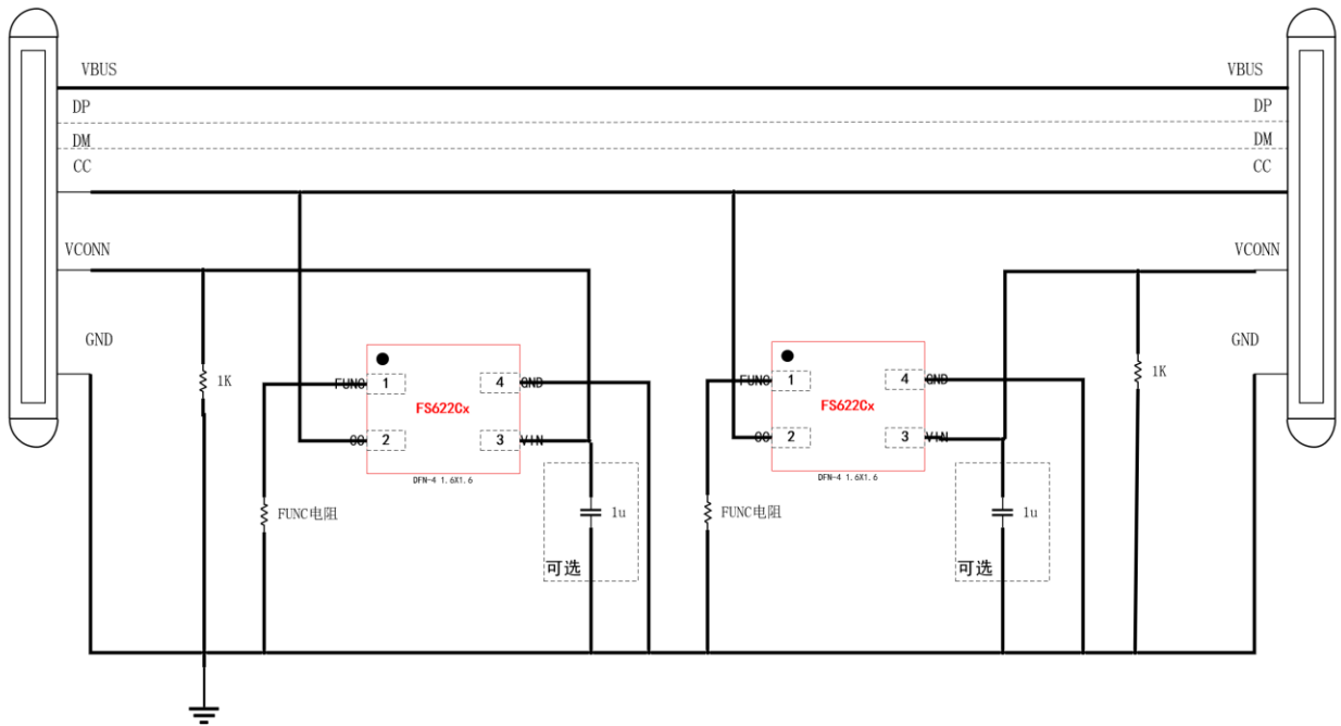
FS622Cx-5芯线双芯片应用图
