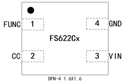
图 1.引脚定义
