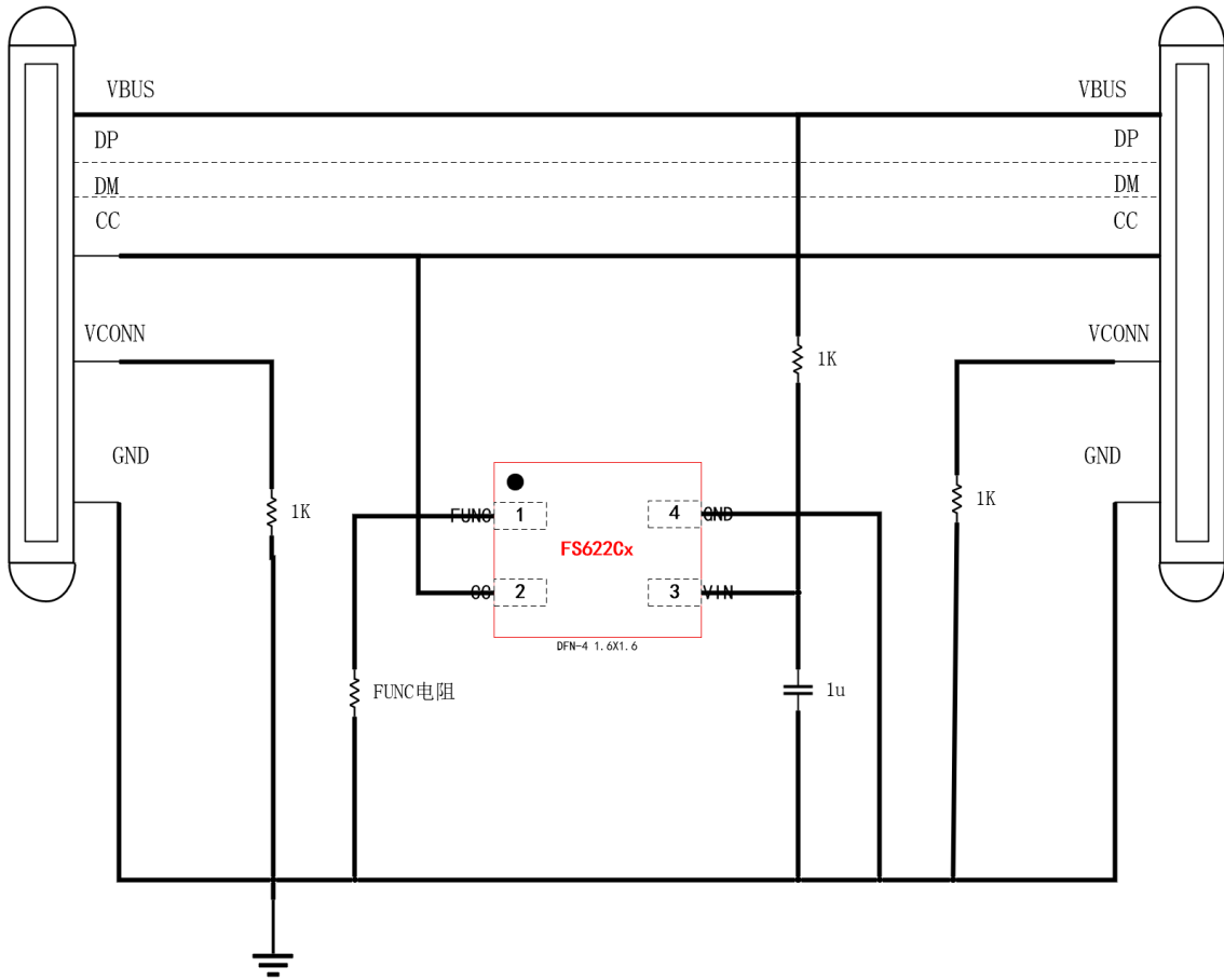
FS622Cx-5芯线单芯片应用图
