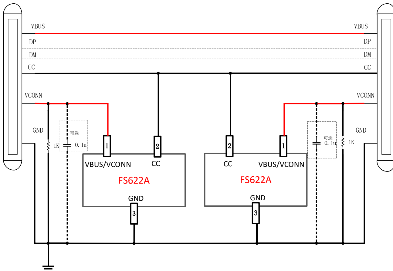
FS622A-5芯线双芯片应用图
