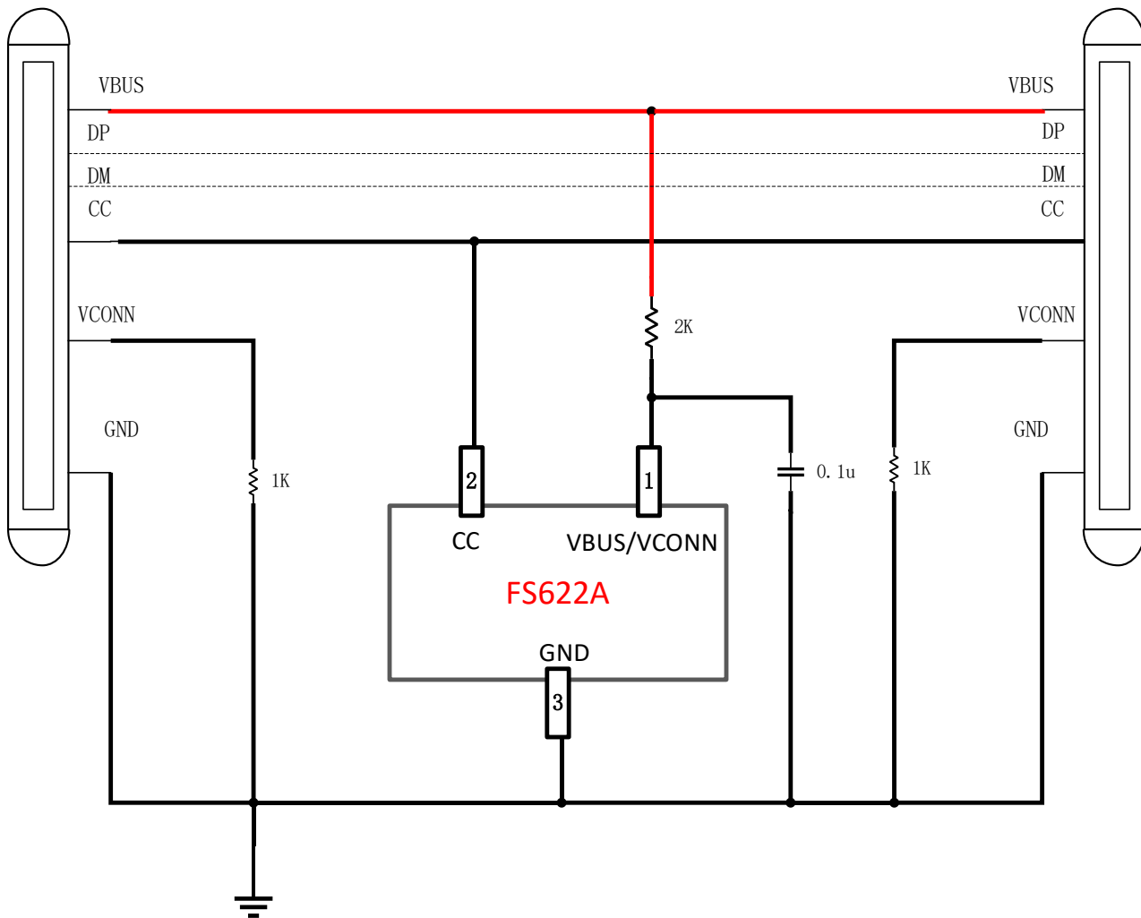
FS622A-5芯线单芯片应用图
