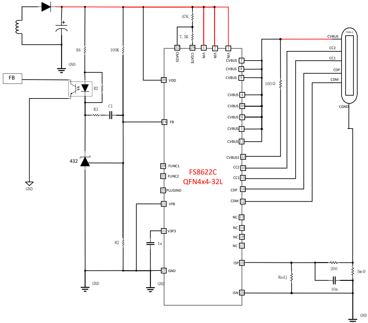
图2.FS8622C 应用图
