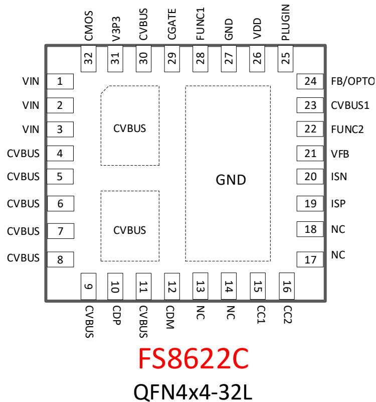
图 1. 引脚定义
