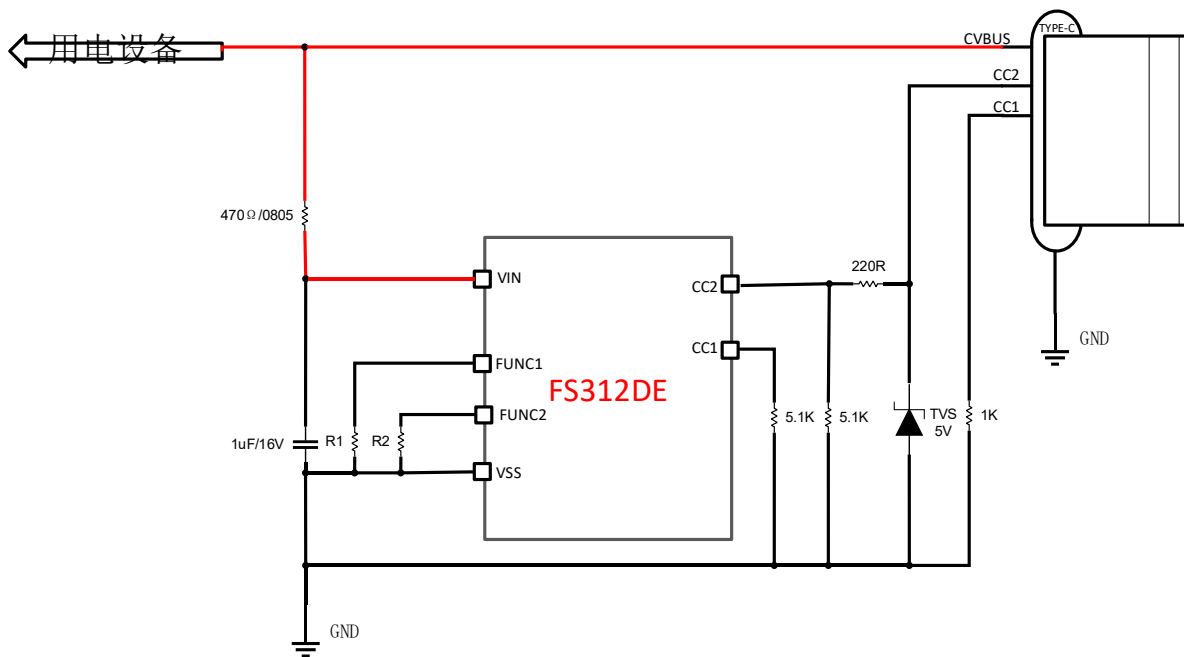
图2. FS312DE 应用图
