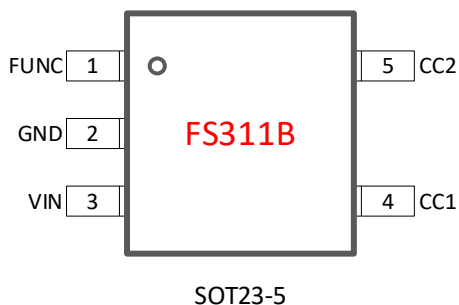
图 1. 引脚定义
