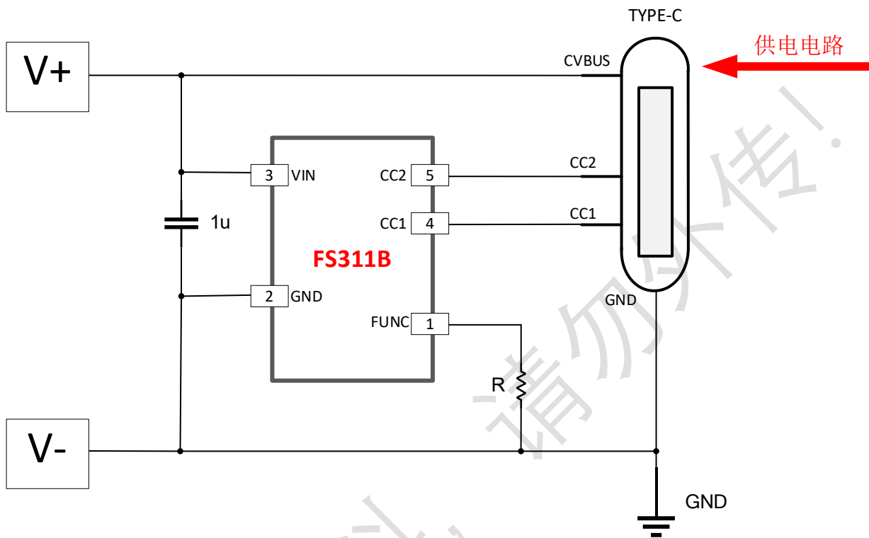
图2. FS311B应用图
