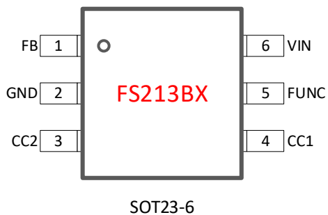
图 1. 引脚定义
