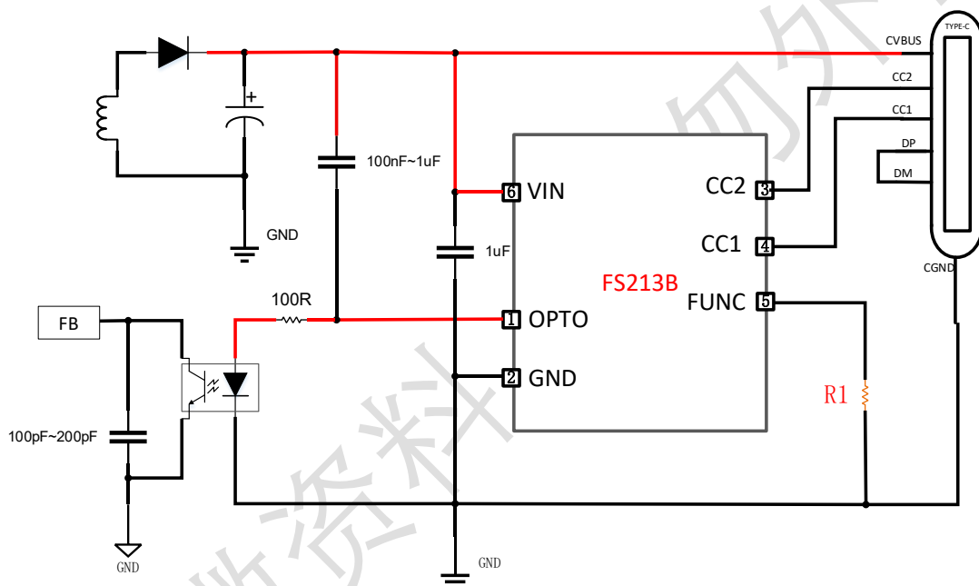
图2. FS213B应用图
