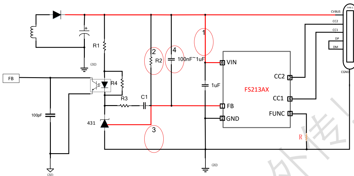
图3. FS213AX模拟MOS应用图
