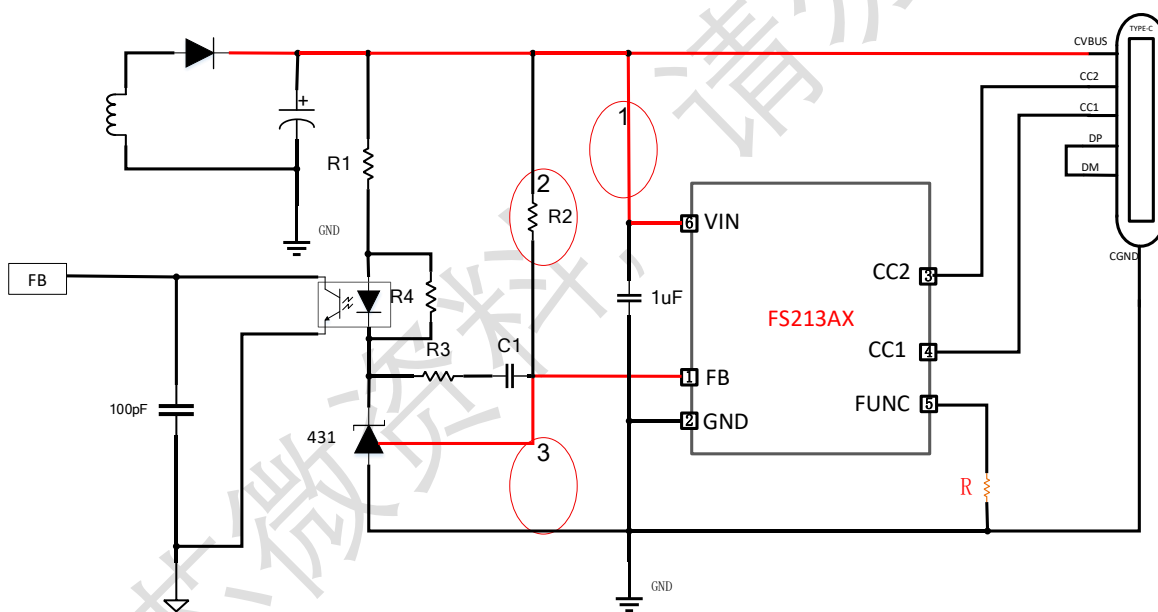
图2. FS213AX直驱光耦应用图
