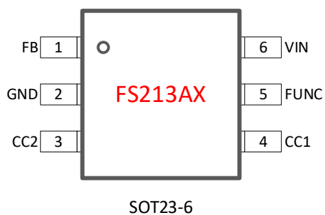
图 1. 引脚定义
