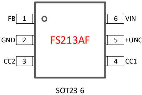
图 1. 引脚定义
