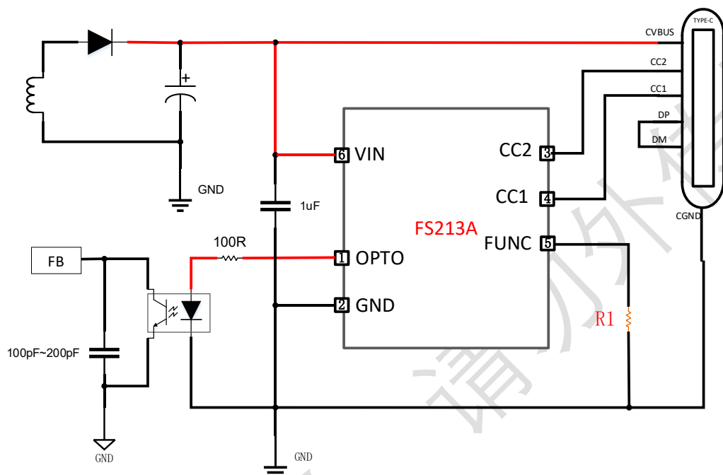
图2. FS213A直驱光耦应用图
