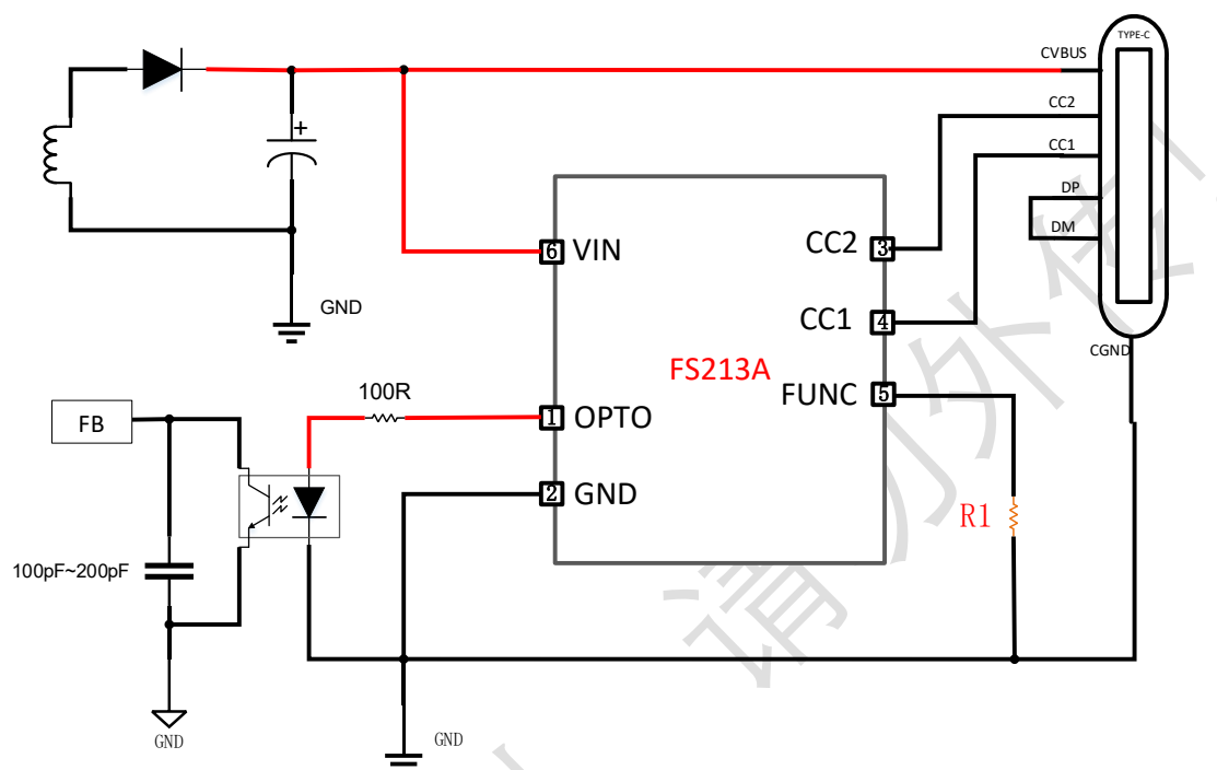
图2. FS213A直驱光耦应用图
