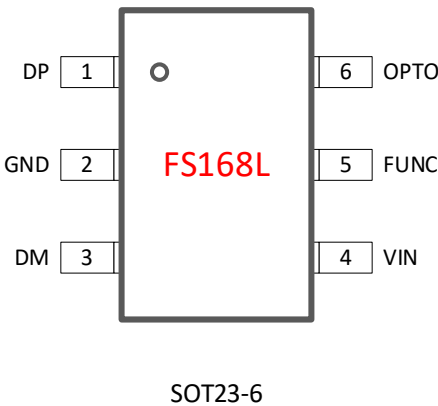
图 1. 引脚定义
