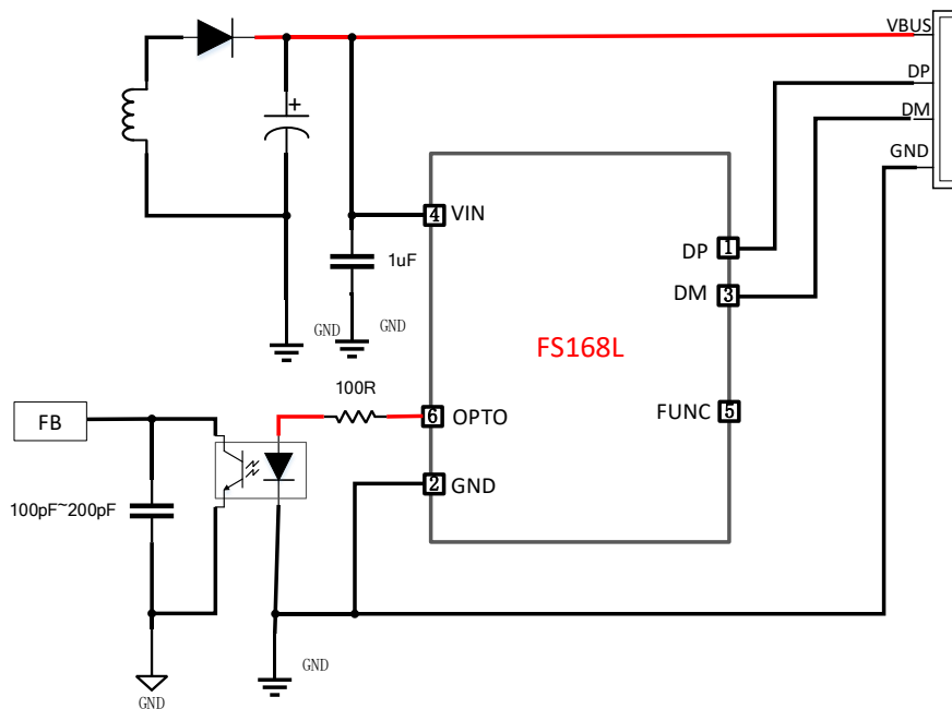
图2. 应用图
