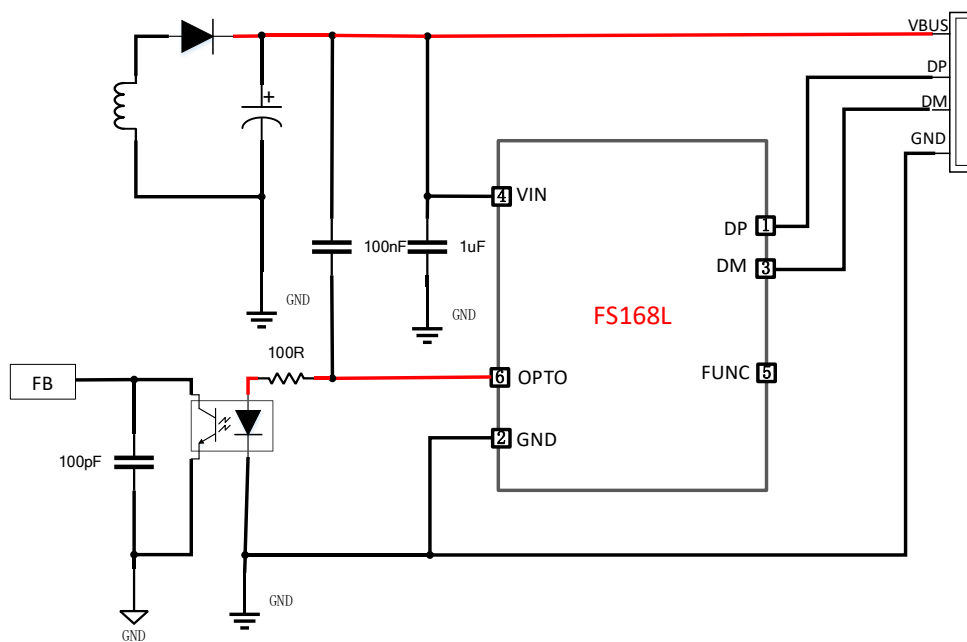
图3. 应用图
