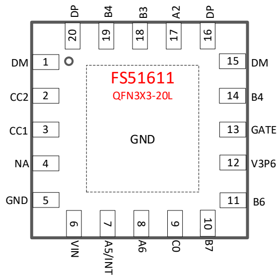
图 1. 引脚定义
