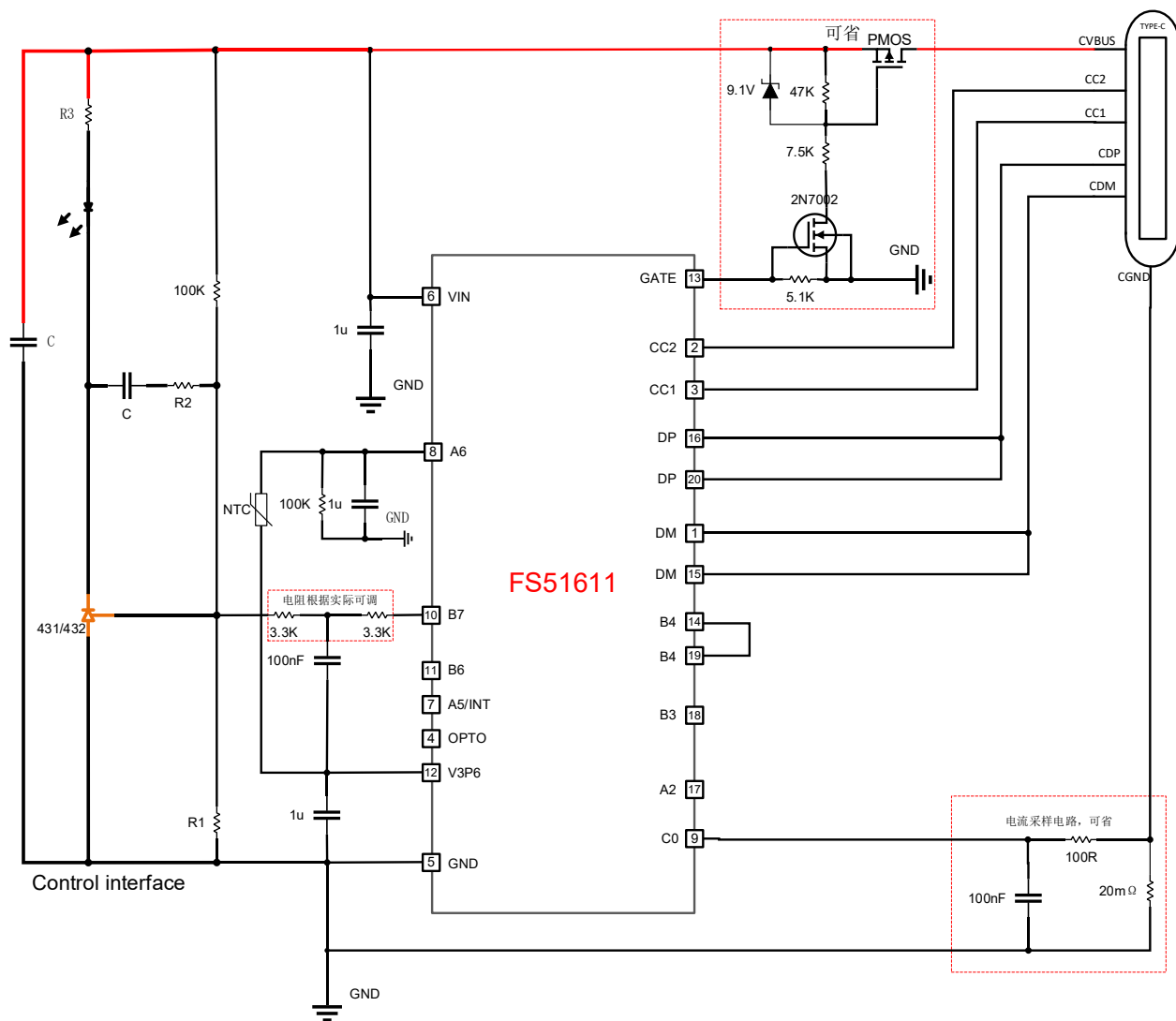
FS51611 应用图
