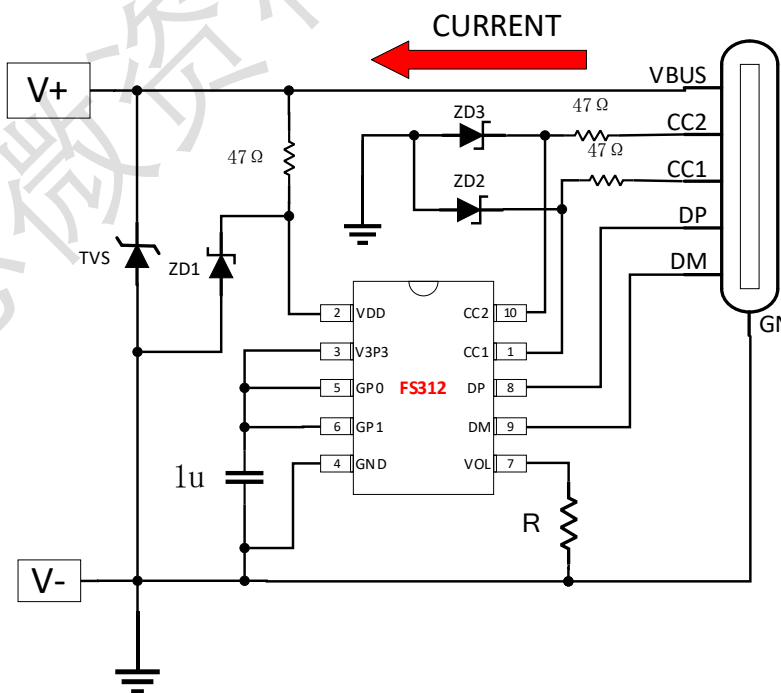
图3.应用图
