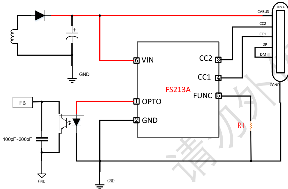
图2. FS213A直驱光耦应用图
