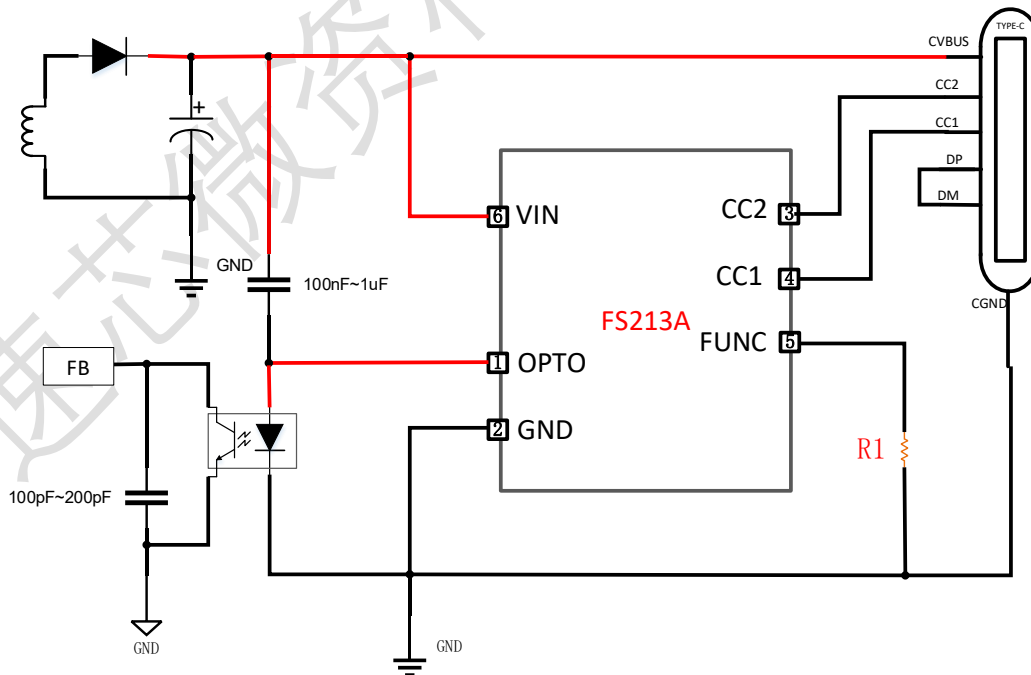
图3. FS213A模拟MOS应用图
