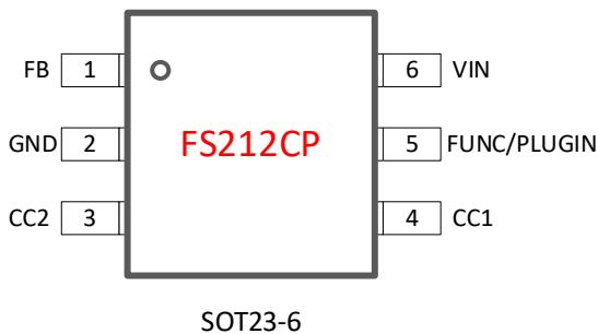
图 1. 引脚定义
