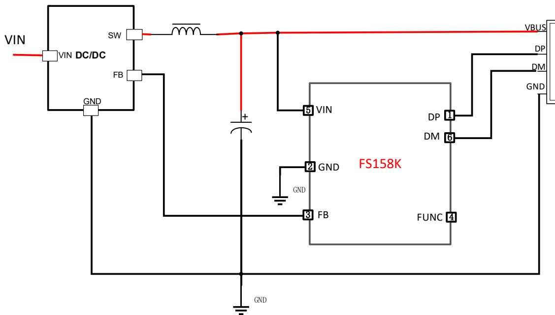
图2. 应用图
