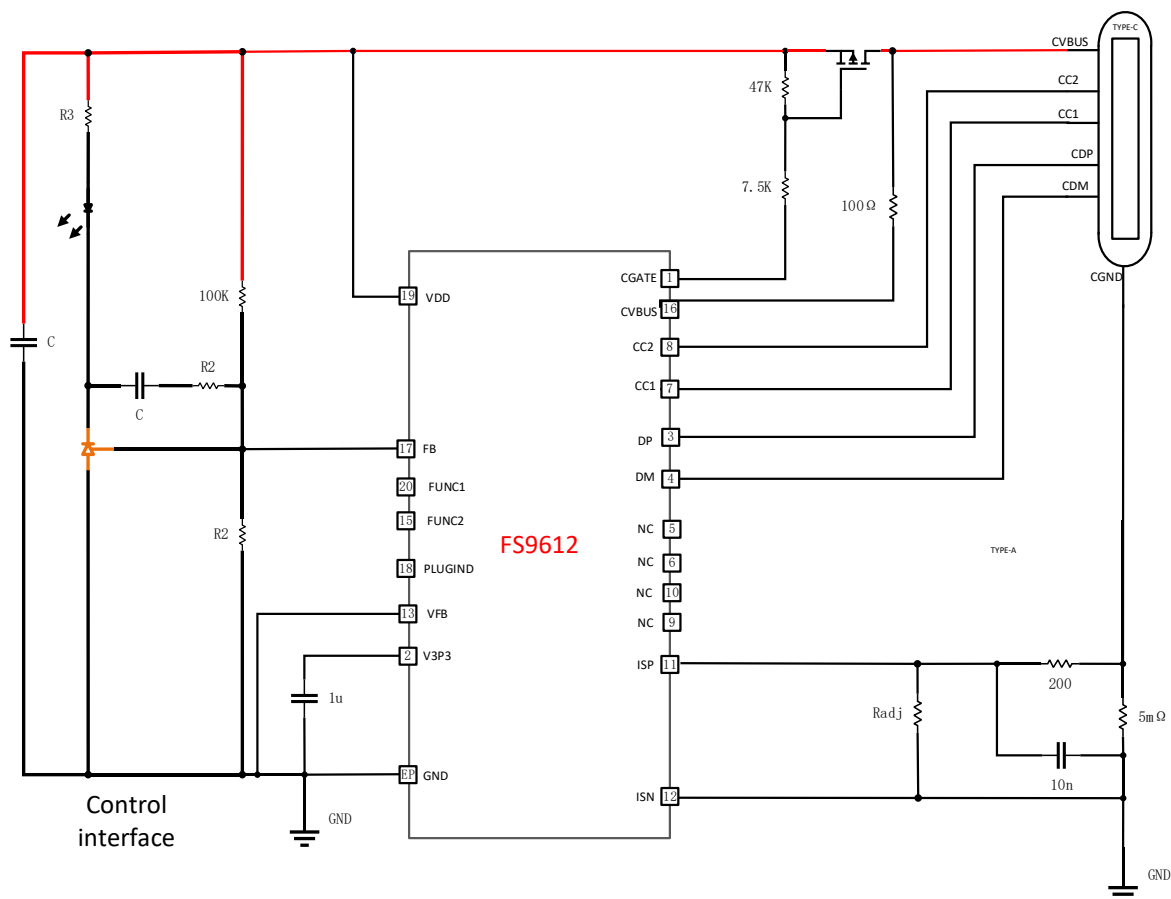
图3.FS9612应用图
