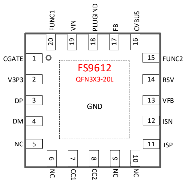
图 1. 引脚定义
