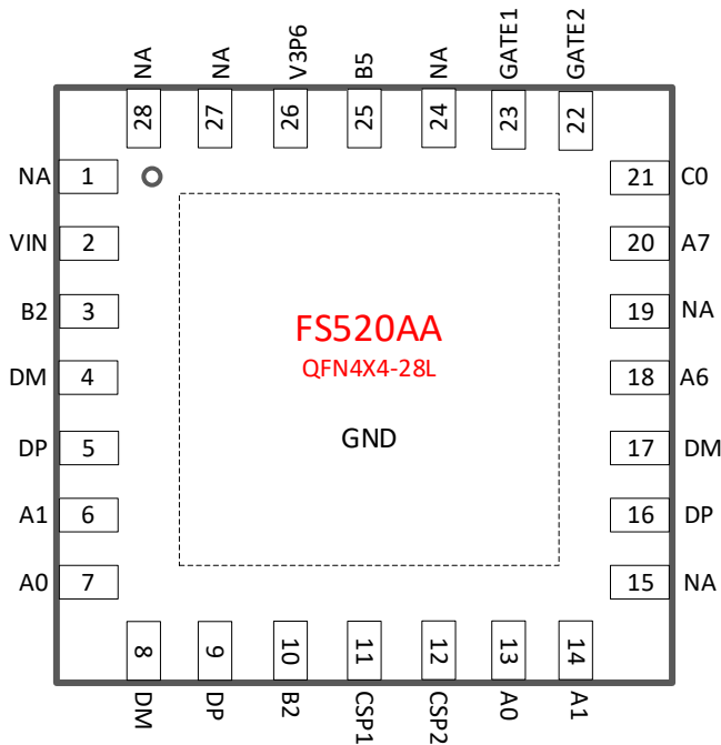
图 1. 引脚定义
