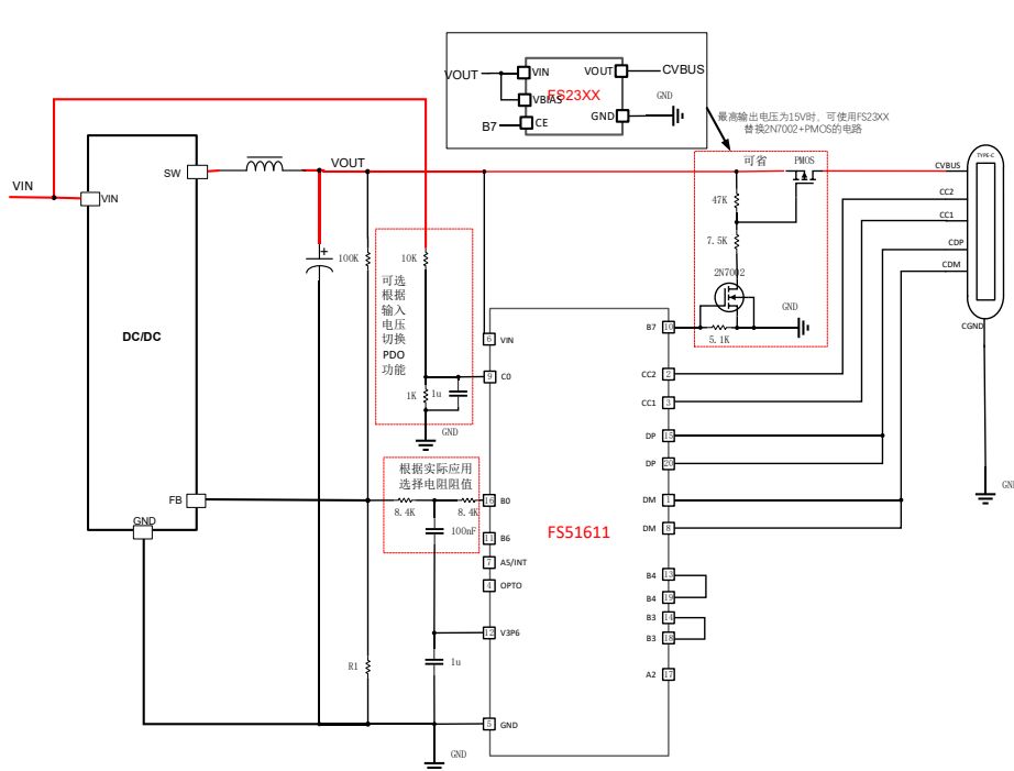
FS51611 车充应用图
