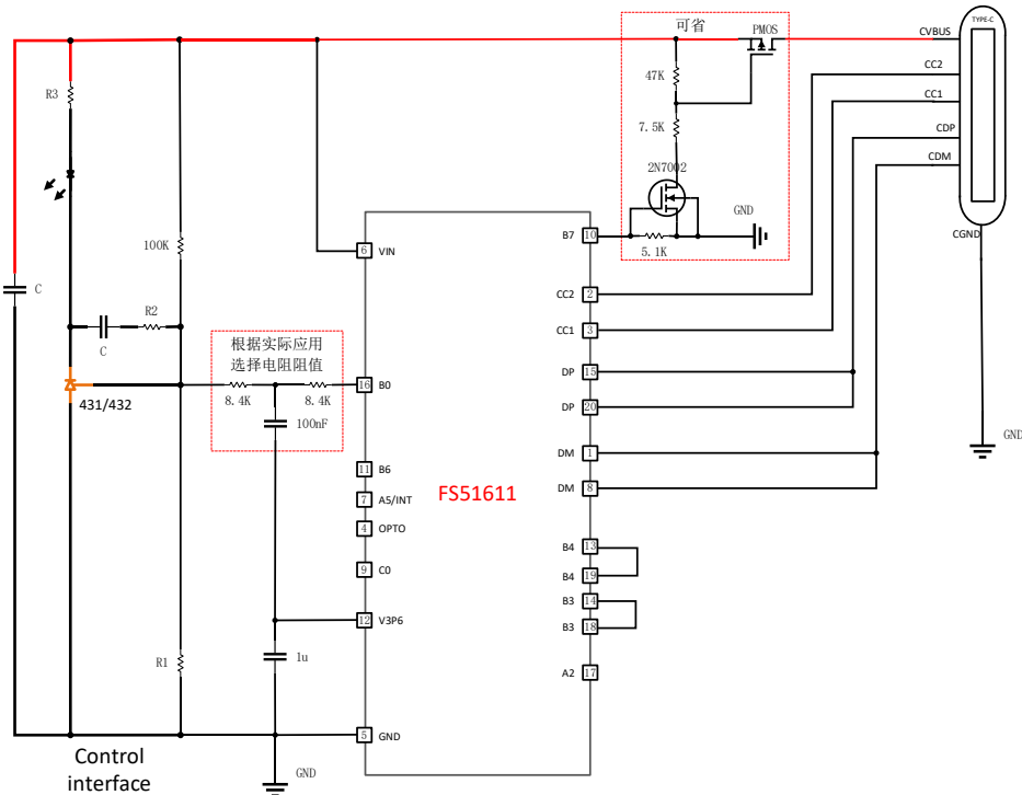
FS51611 功率140W最高28V以下的应用图
