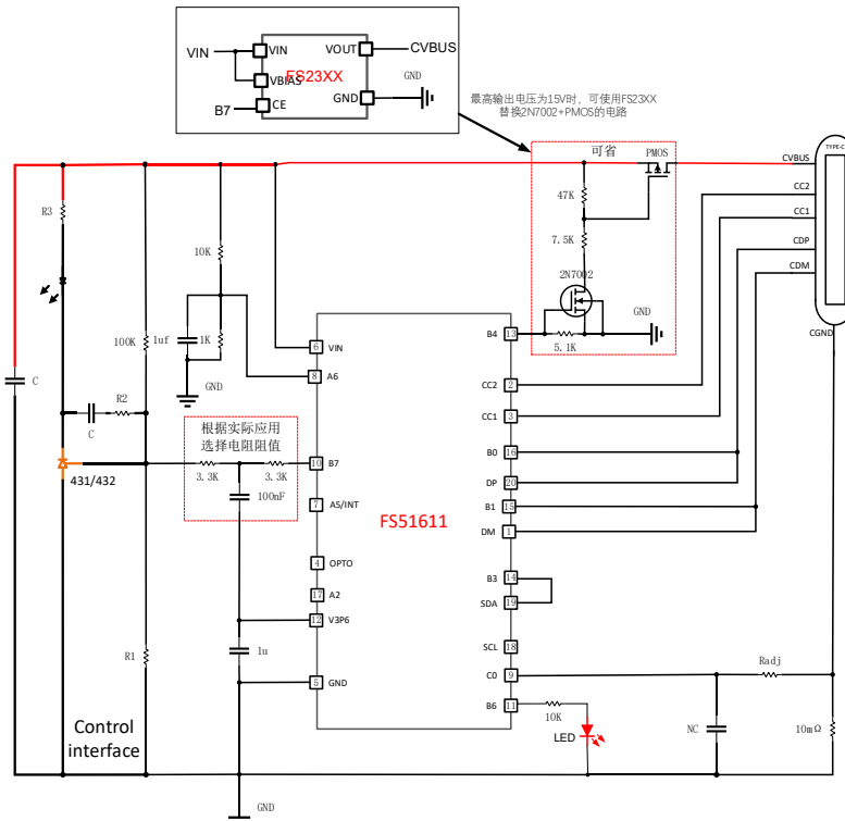
FS51611 输出电压最高28V且带快充指示的应用图
