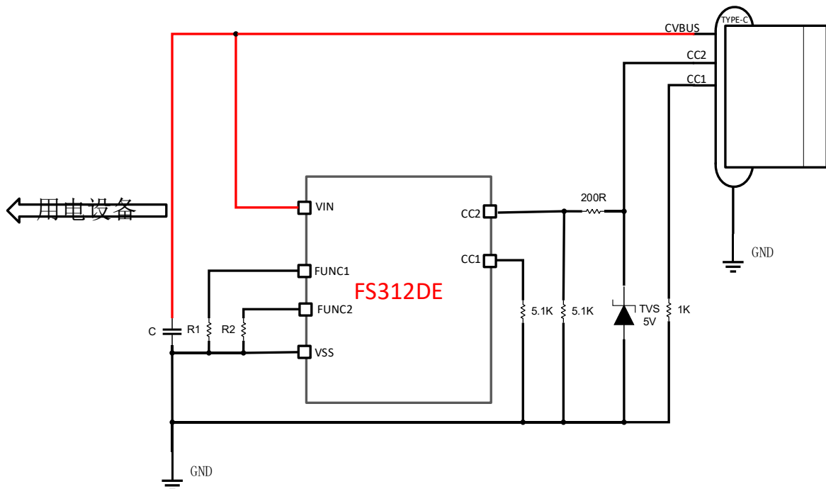
图2. FS312DE 应用图
