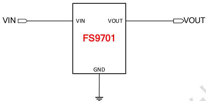
图4. 应用图
