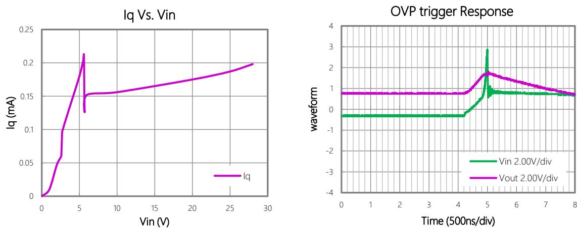
图3. FS9701特性曲线图
