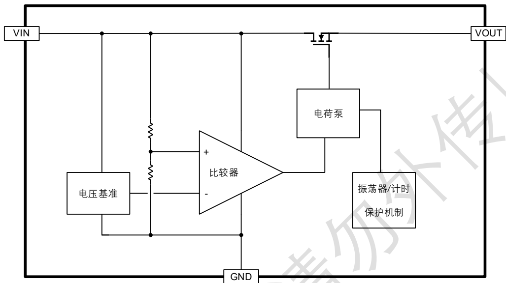
图2. FS9701内部框图
