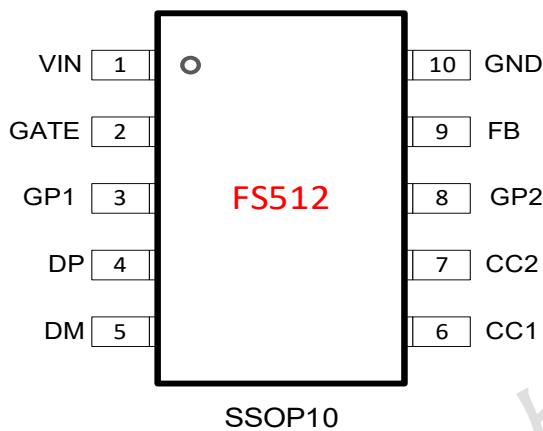
图 1. 引脚定义
