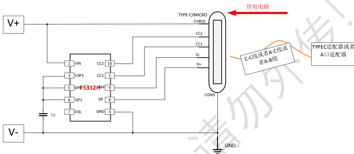
图2. 应用图
