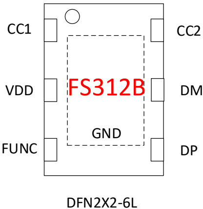
图 1. 引脚定义
