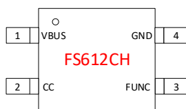
SOT143
