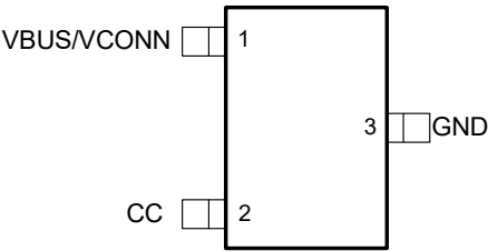
图 1.引脚定义
