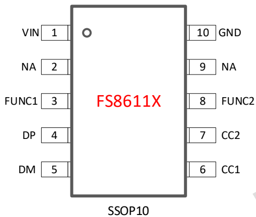
图 1. 引脚定义
