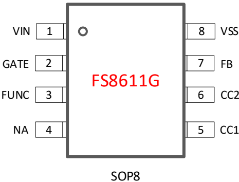
图 1. 引脚定义
