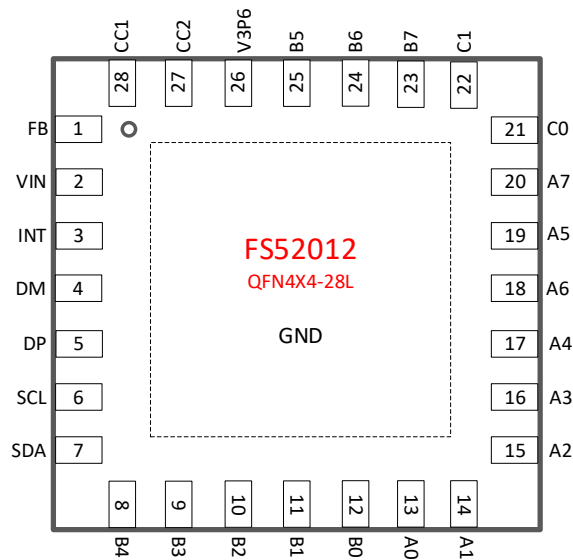
图 1. 引脚定义
