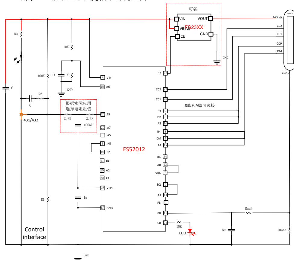
FS52012 功率140W最高28V以下且带快充指示的应用图
