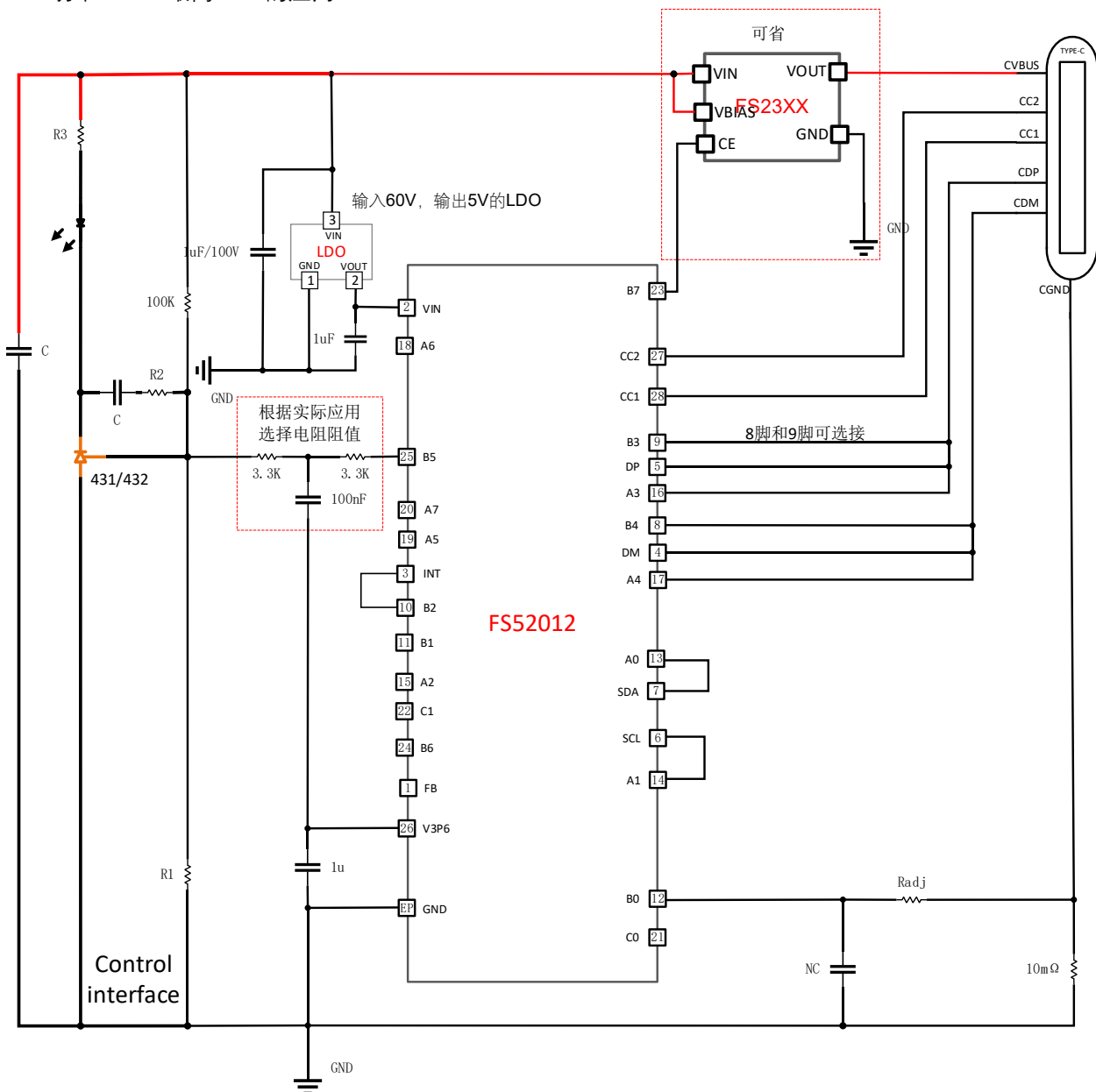
FS52012 240W最高48V应用图
