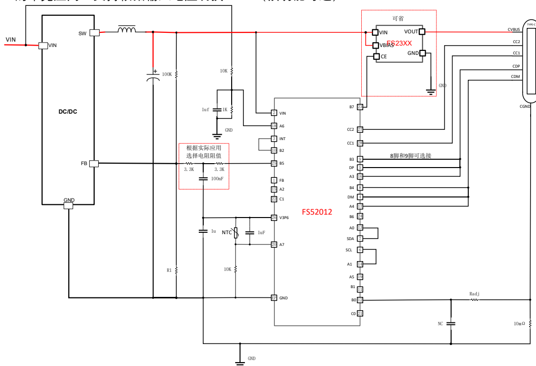
FS52012 车充应用图
