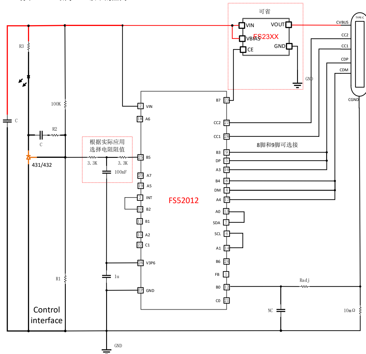
FS52012 功率140W最高28V以下的應用图
