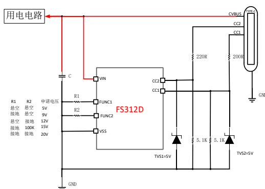
图 3FUNC 脚固定应用图
