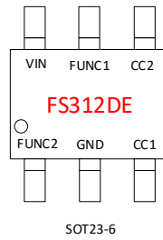
图 1. 引脚定义
