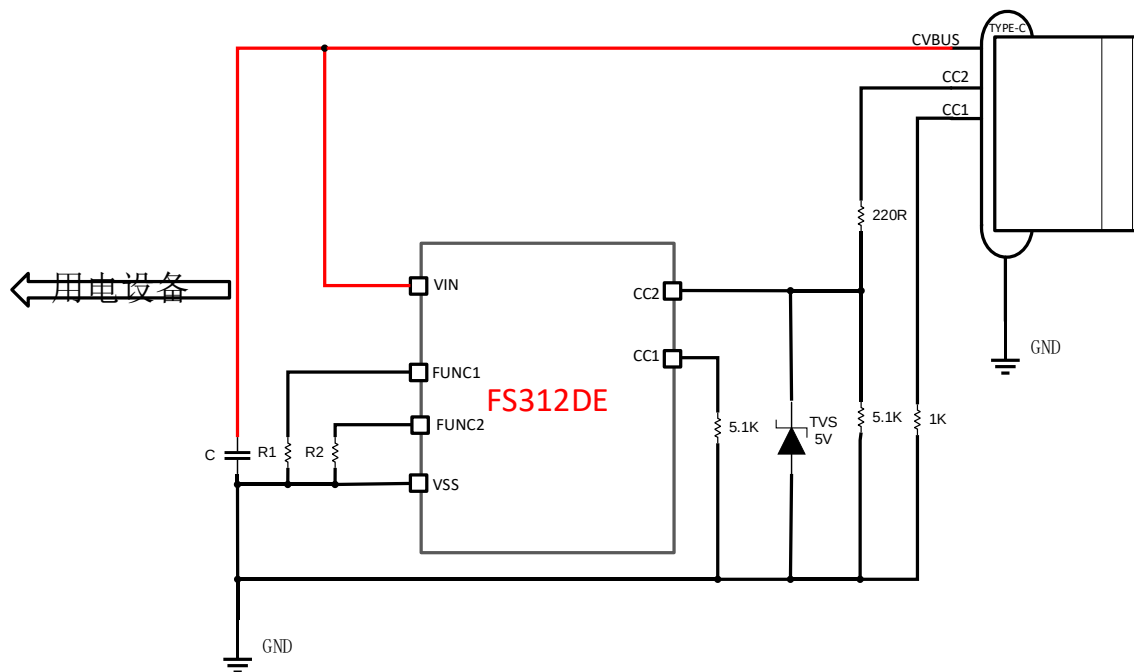
图2. FS312DE 应用图
