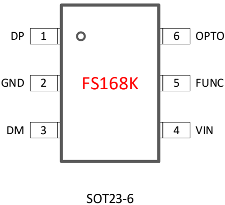
图 1. 引脚定义
