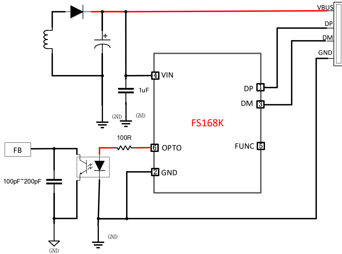
图2. 应用图
