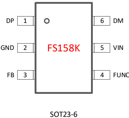
图 1. 引脚定义
