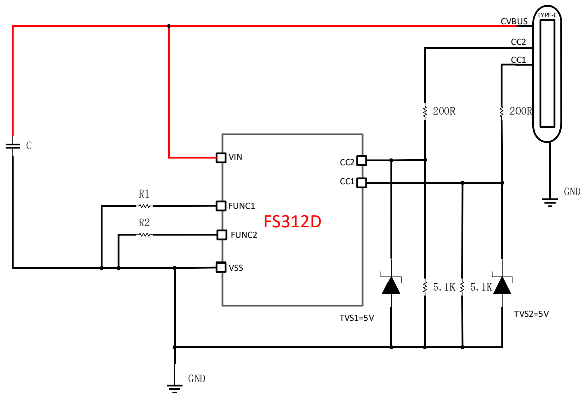
图2. FS312D 应用图
