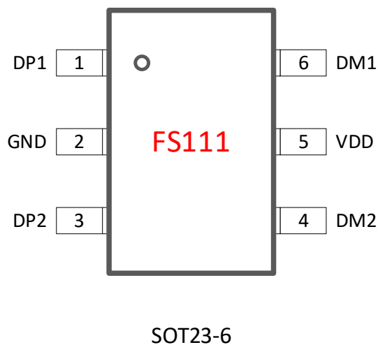
图 1. 引脚定义
